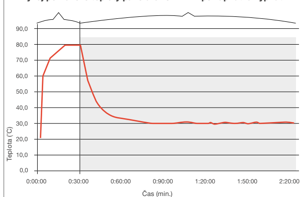
Vývoj povrchové teploty panelu GLOA 2 kW po zapnutí a vypnutí
